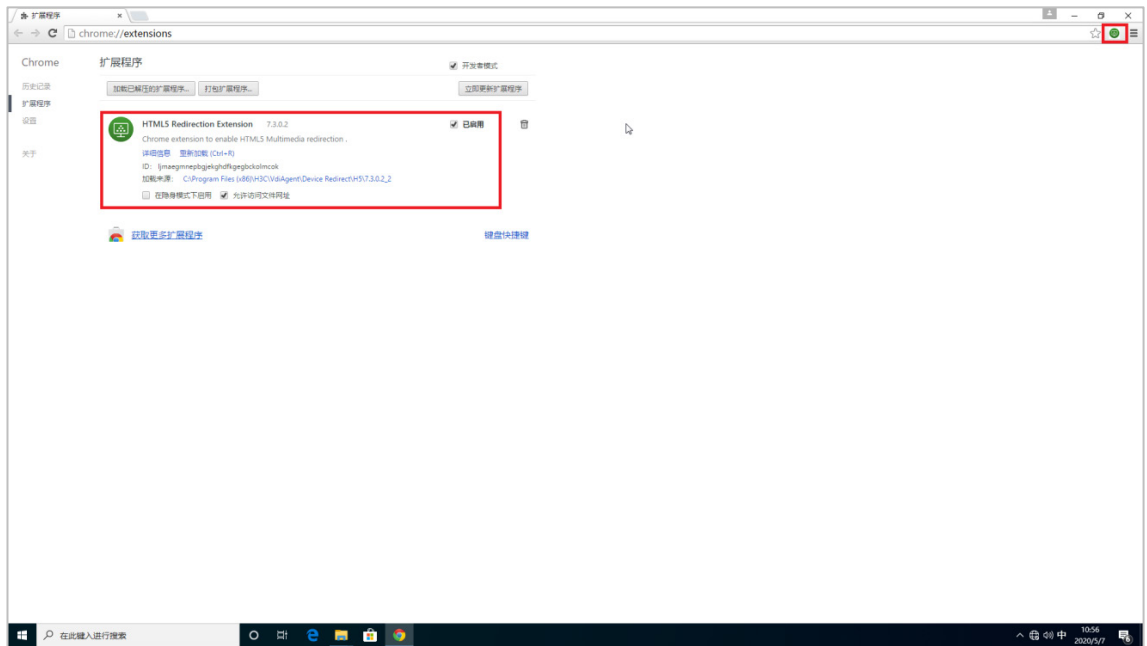
图4-10 加载成功
