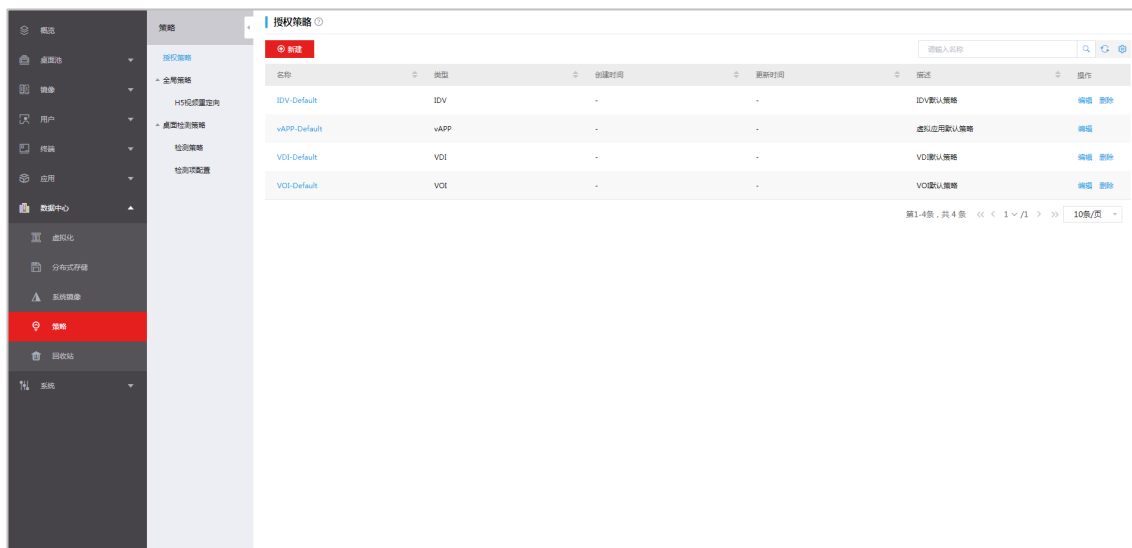
图3-1 授权策略
