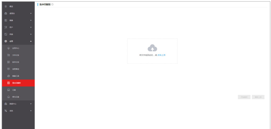
图3-4 盲水印解析
