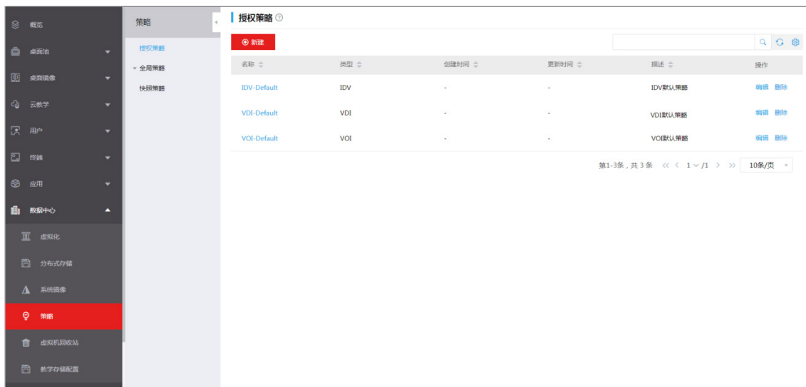
图3-1 授权策略
