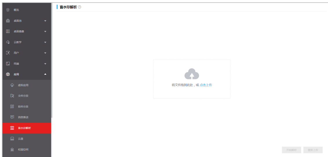
图3-4 盲水印解析
