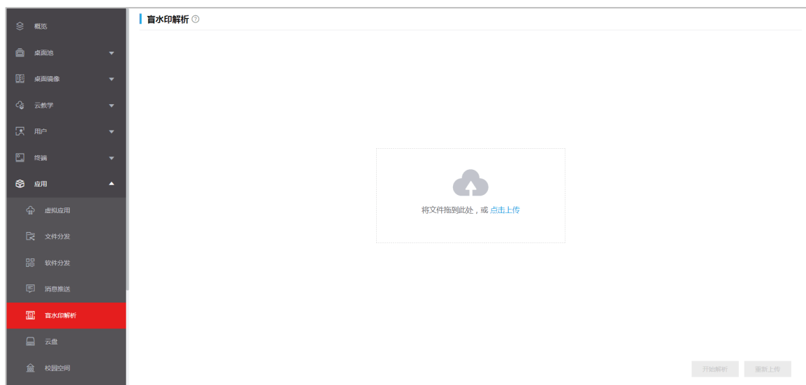
图5 盲水印解析
