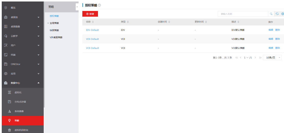
图2 授权策略
