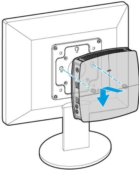
图2-5 安装云终端
